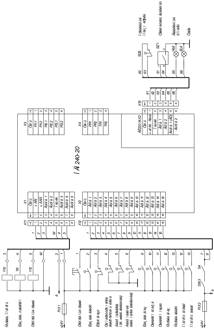
Схема подключения ОГМ240-20 для КС-55722-2
