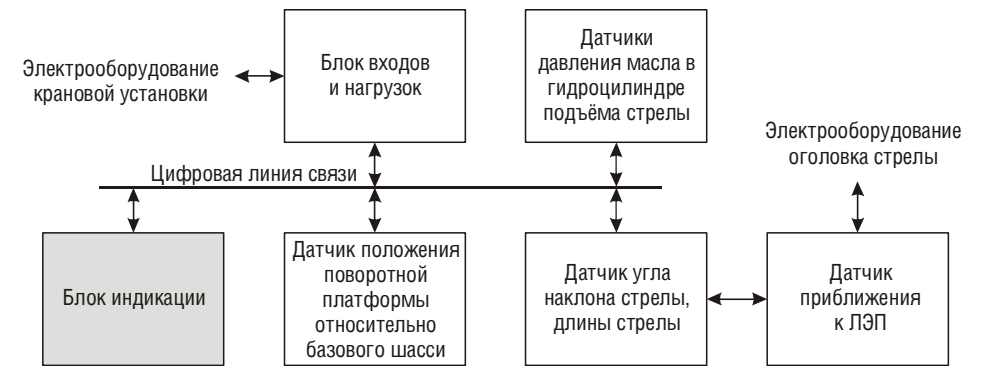
Рисунок 1 — Структурная схема ОГМ240
