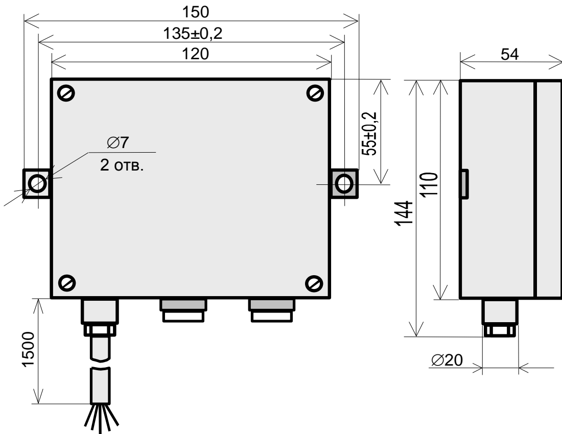
Рисунок 9 - Габаритные и присоединительные размеры БР
