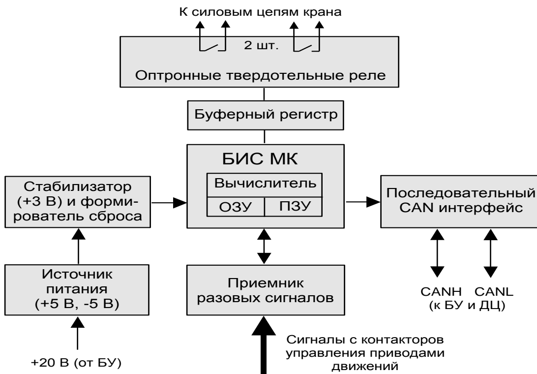
Рисунок 6 - Блок-схема БР
